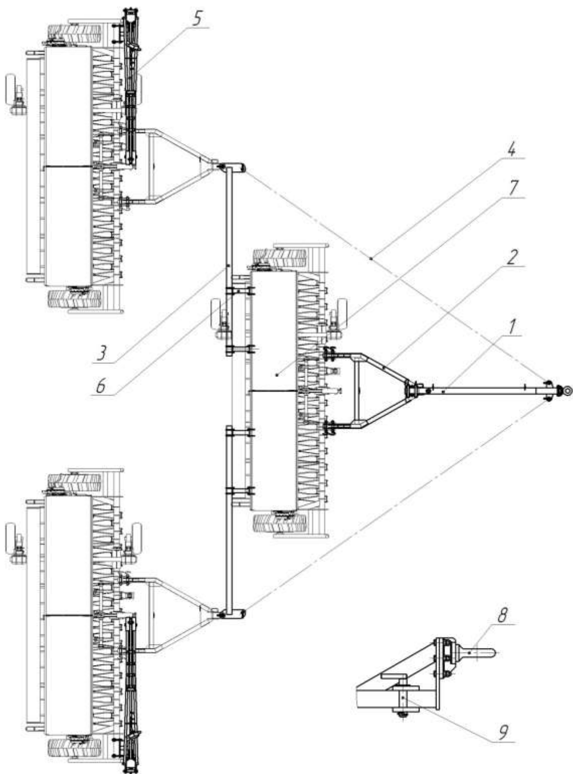
Рис. 1. Широкозахватный посевной агрегат УС-3 + 3хЗС-42
