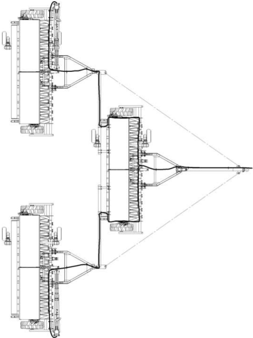
Рис. 6. Схема расположения РВД гидропривода маркеров
